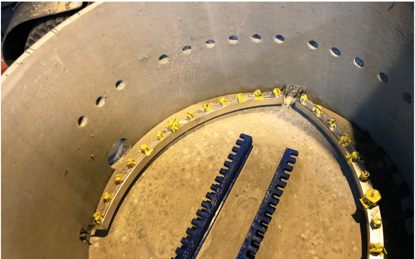
Eksempel på løsning med kjerneboring \varnothing 53 mm + AR-32 pakning for hver stikkledning
