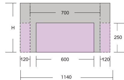
Kortside
